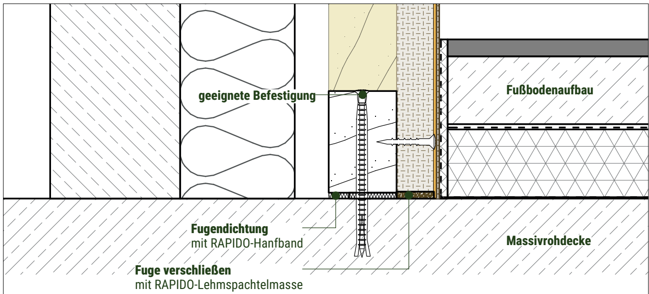
Anschluss Massivboden
