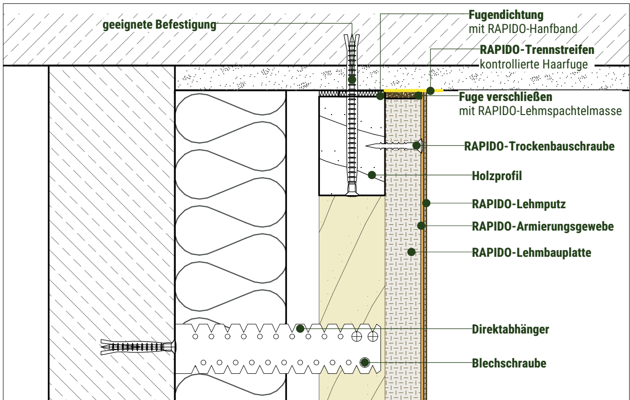
Anschluss Massivdecke
